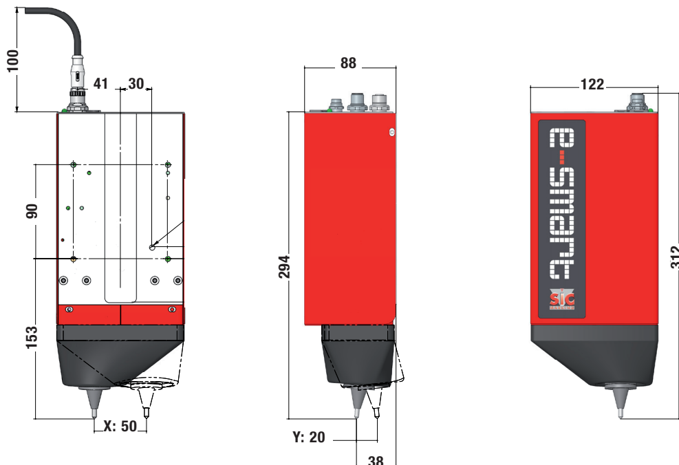
Área de marcado-50 x 20 mm
